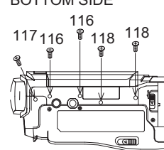
BOTTOM SIDE
