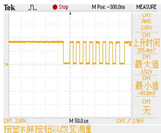
图7. XP11.9 AMP_SCL
