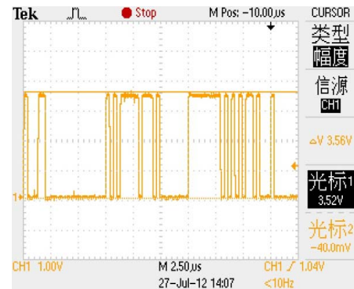
图3. XP11. 3 DATA1
