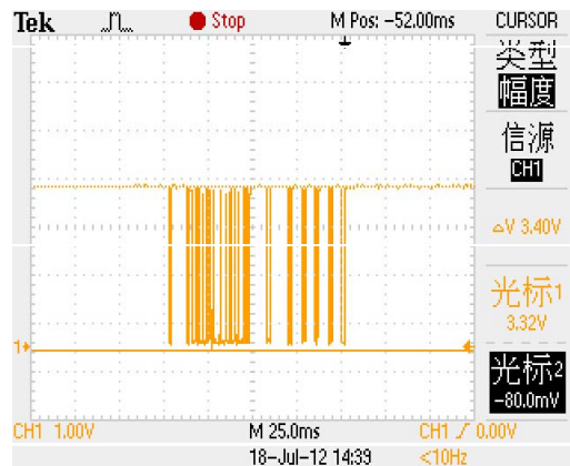
图8. XP11.10 AMP_SDA
