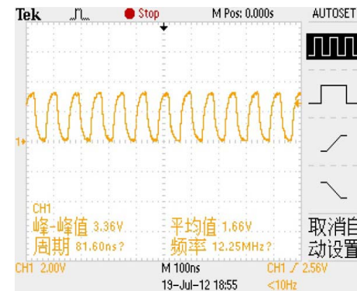
图6. XP11. 7 MCLK
