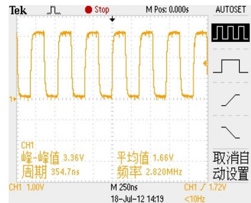
图5. XP11. 5 BCLK
