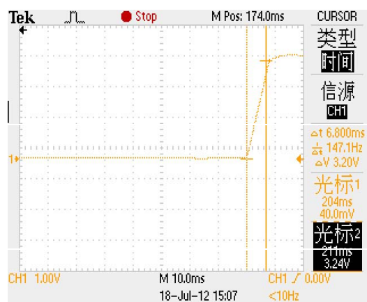
图10. XP11.13 AMP_RST
