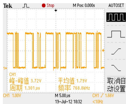
图1. XP11. 1 DATA0
